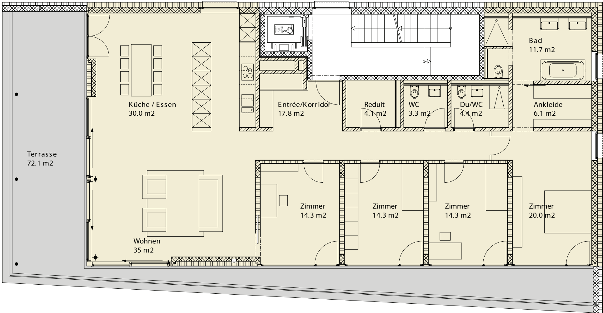
1.Obergeschoss Haus 23 BGF 215.2 m 2
